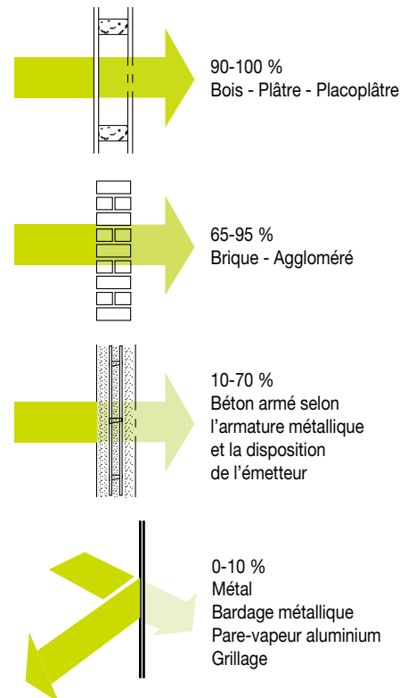
Influence d'un obstacle sur la transmission radio
