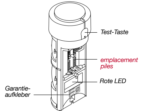
Erfassungsmodul, Rückseite
