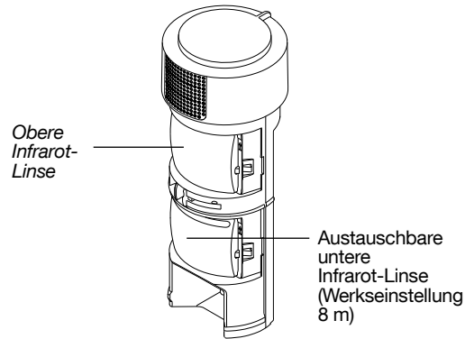
Erfassungsmodul, Vorderseite
