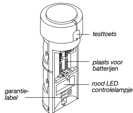
Detectiemodule achterkant
